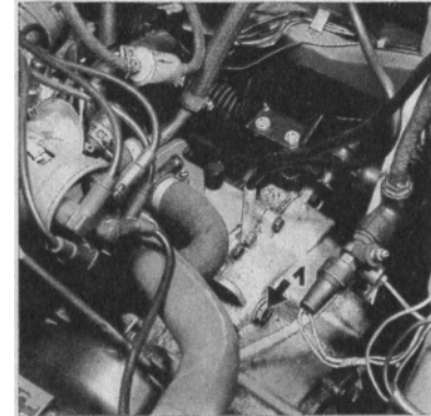
Bild 41. Getriebe (1) Öleinfüllschraube
