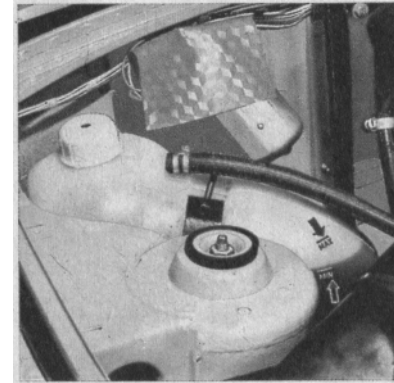
Bild 37. Ausgleichsbehälter
