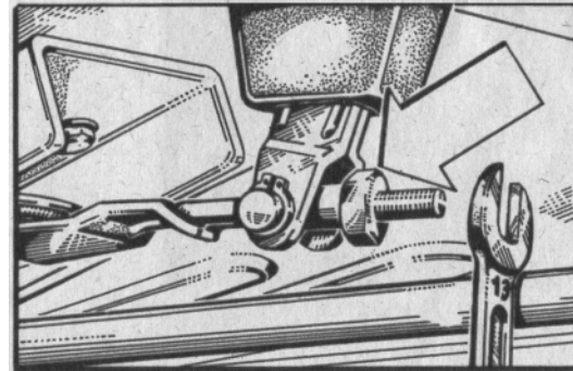
Bild 39. Handbremse nachstellen
